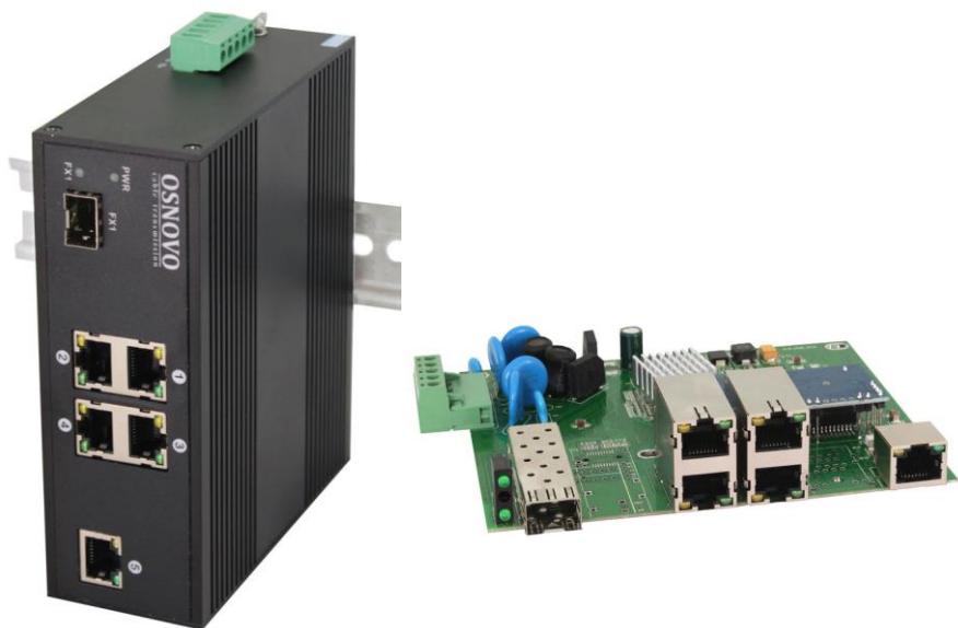
Рис.1 Коммутаторы SW-40501/IC, SW-40501/IC-P , внешний вид
