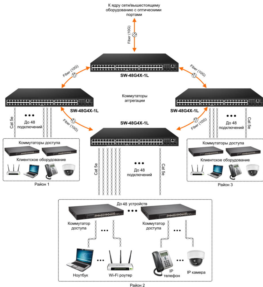
Рис. 8 Схема подключения на примере построения системы видеонаблюдения на предприятии с использованием SW-48G4X-1L
