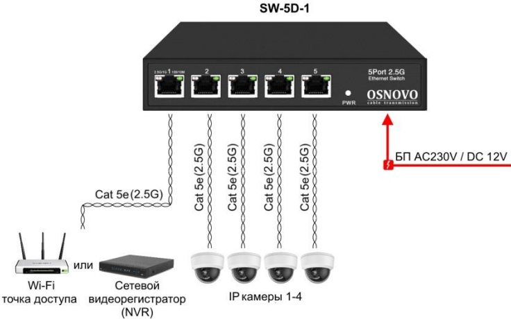
Рис.4 Типовая схема подключения коммутатора SW-5D-1
