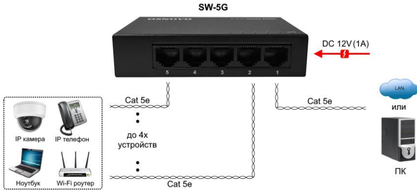
Рис. 4 Типовая схема подключения коммутатора SW-5G.
