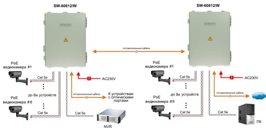
Рис.7 Схема каскадного подключения коммутатора SW-60812/W
