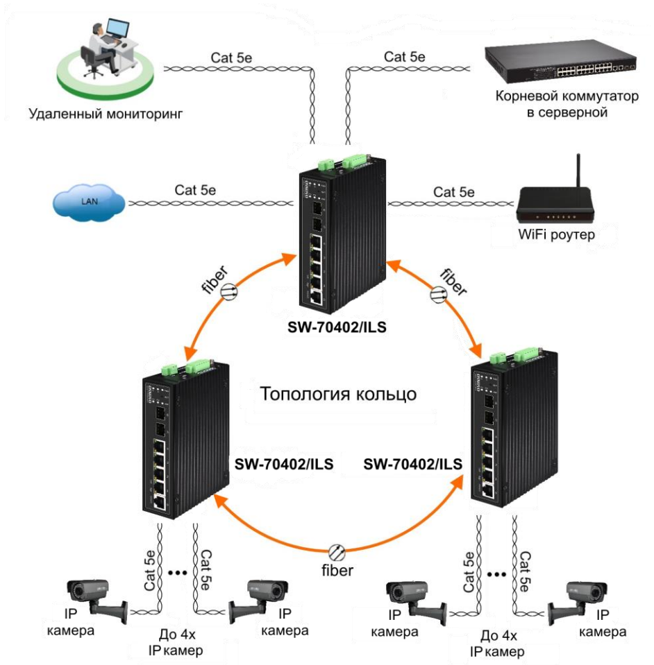
Рис. 10 Схема подключения коммутатора в топологии «кольцо» на примере SW-70402/ILS
