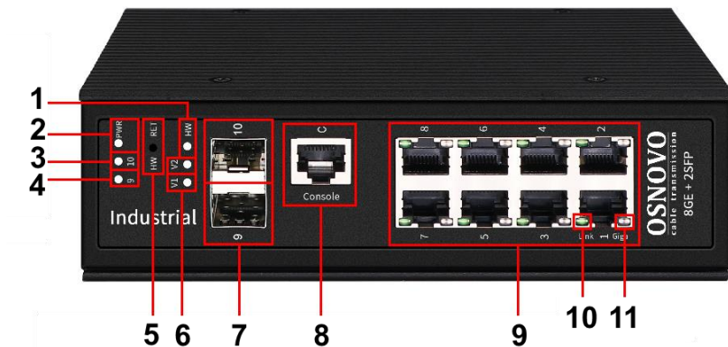
Рис.5 Коммутатор SW-70802/ILS, разъемы, кнопки и индикаторы на передней панели
