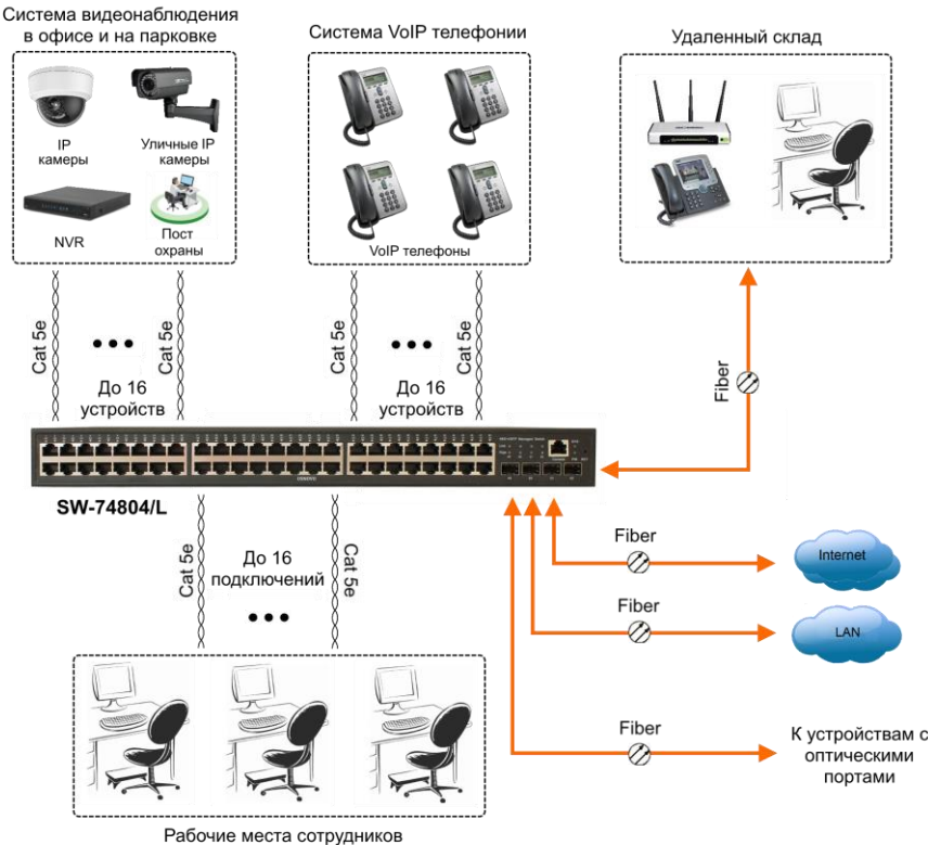
Рис. 3 Схема подключения коммутатора SW-74804/L на примере сети для большого разветвленного офиса
