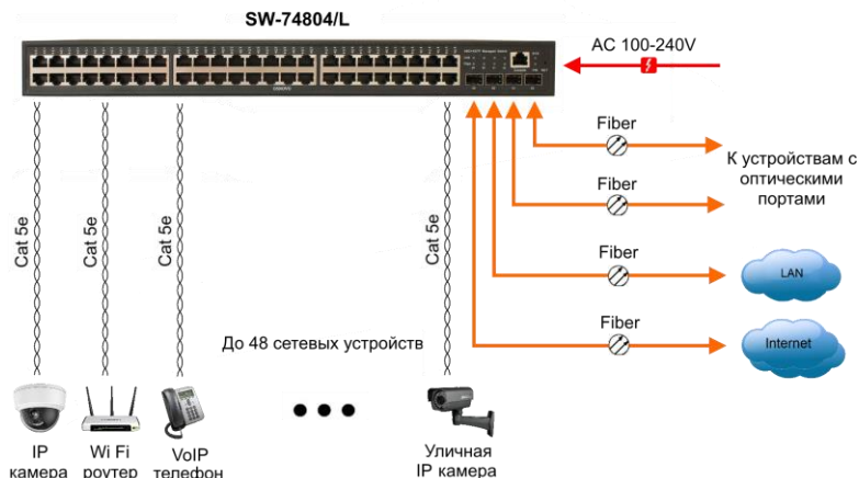
Рис. 4 Типовая схема подключения коммутатора SW-74804/L
