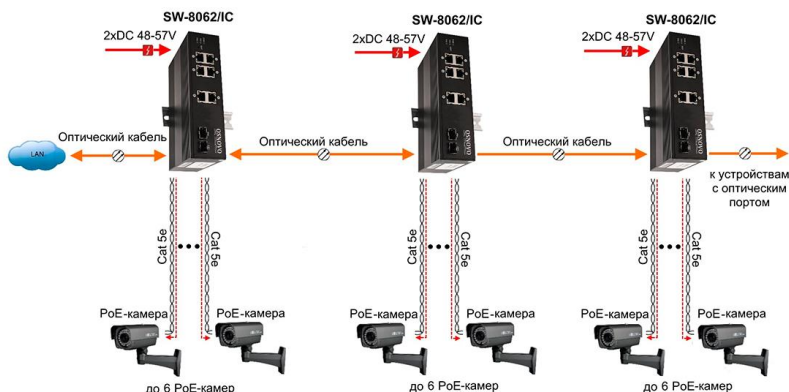
Рис.4 Типовая схема подключения коммутатора SW-8062/IC
