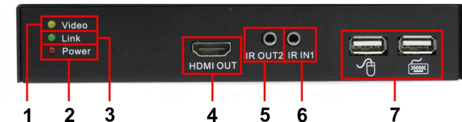
Рис. 4 Приемник RA-HiKM, разъемы и индикаторы на передней панели
