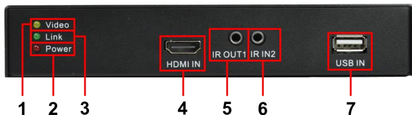
Рис. 2 Передатчик TA-NiKM, разъемы и индикаторы на передней панели
