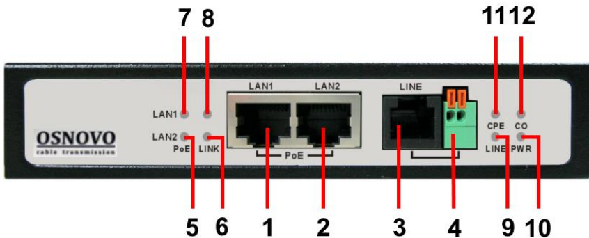
Рис.2 Разъемы и индикаторы удлинителя TR-IP2PoE (передняя панель).
