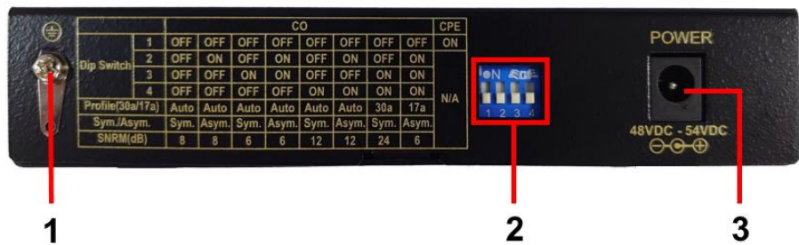
Рис.3 Разъемы и переключатели удлинителя TR-IP2PoE (задняя панель).
