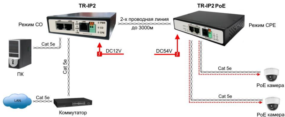
Рис.5 Типовая схема подключения удлинителя TR-IP2PoE
