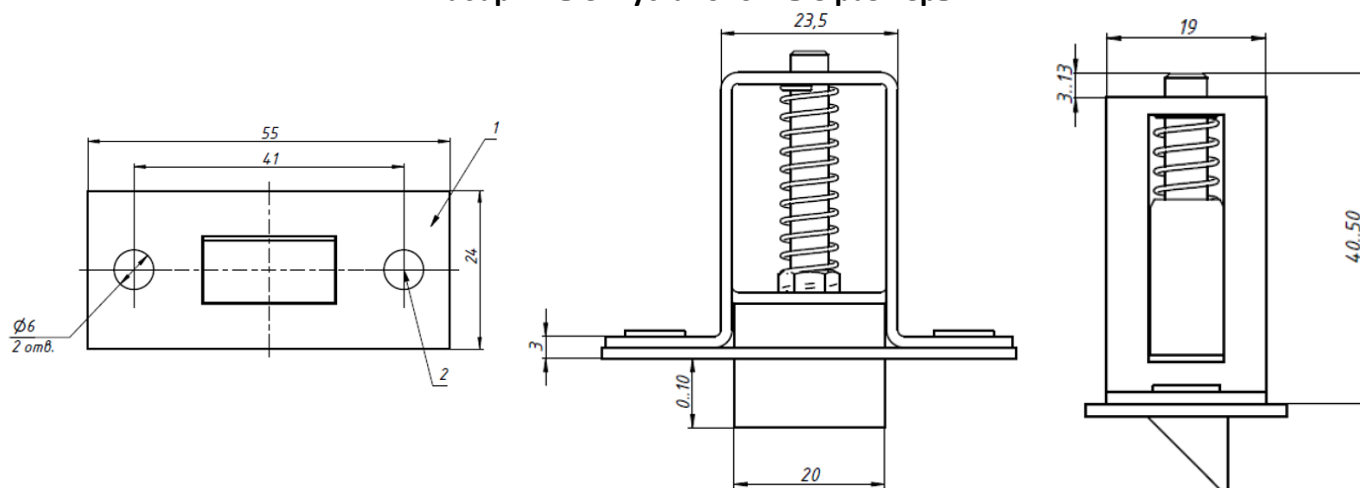
Внешний вид
