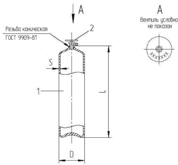
Рис. 2. Общий вид баллона 1-баллон, 2-вентиль, В-дiameter баллона, S-толщина стенки
