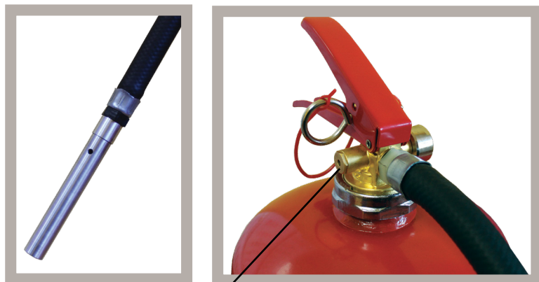
Предохранительный клапан
