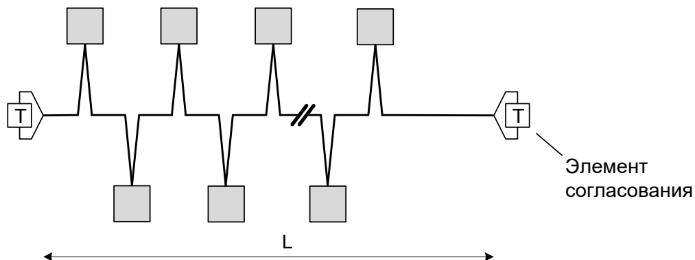
Рисунок 8 Шина без отводов
