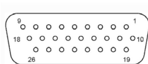
Рисунок 3 – Распиновка разъема на ответной части
