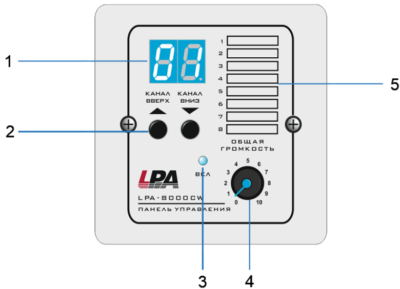
Рис.2. Передняя панель
