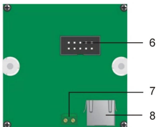
Рис.3 Задняя панель
