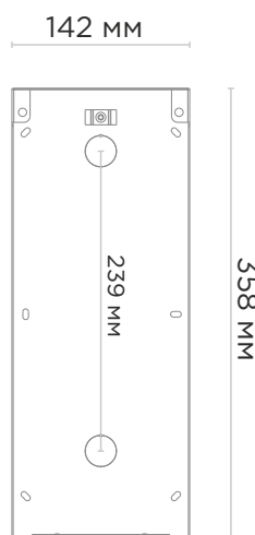
Крепеж для врезного монтажа
