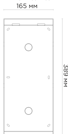
Кронштейн для накладного монтажа с защитным козырьком от солнца и дождя
