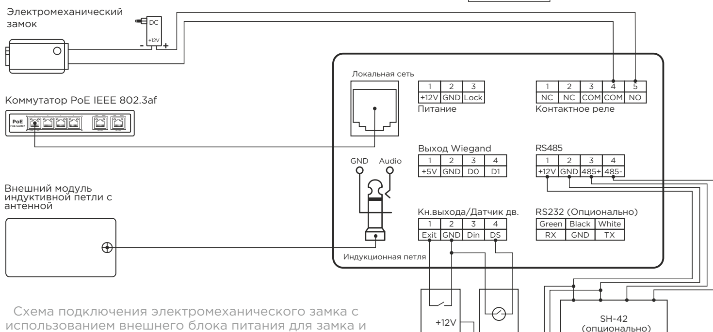
Схема подключения электромеханического замка с использованием внешнего источника питания для замка
