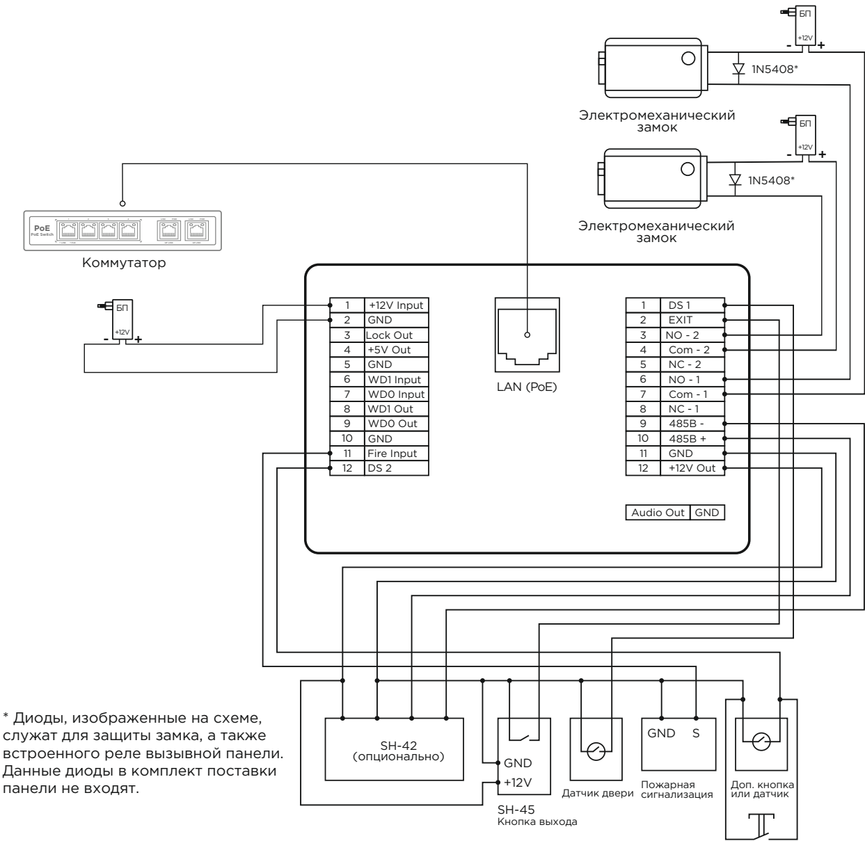
Схема 7. Подключение двух электромеханических замков с использованием встроенных реле панели и отдельных блоков питания для замков и панели.
