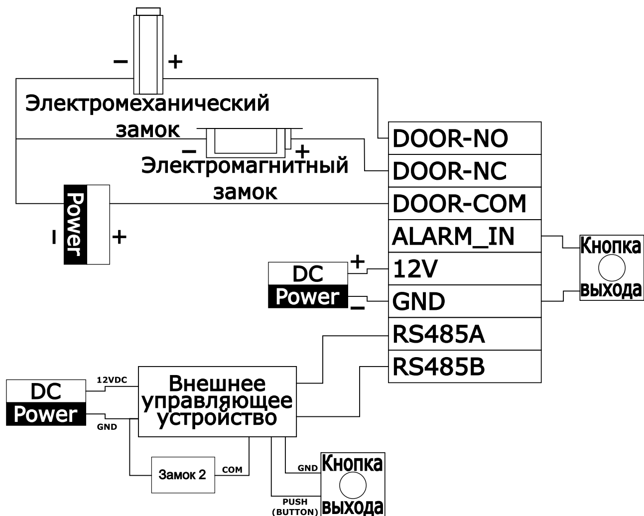
Рисунок 3.5 – Схема подключения. Замок 2
