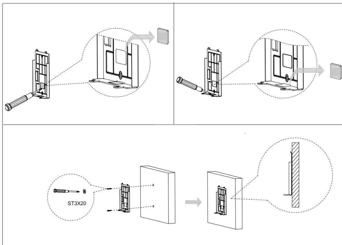
Рисунок 4.6 – Схема установки
