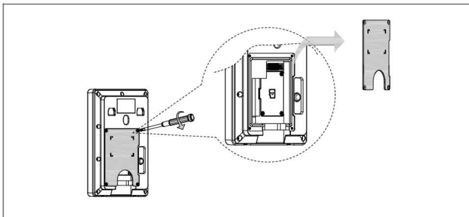
Рисунок 4.3 – Установка карты
