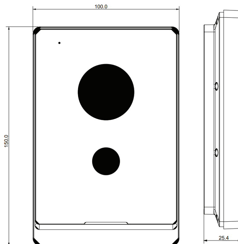
Рисунок 4.1 – Габаритные размеры
