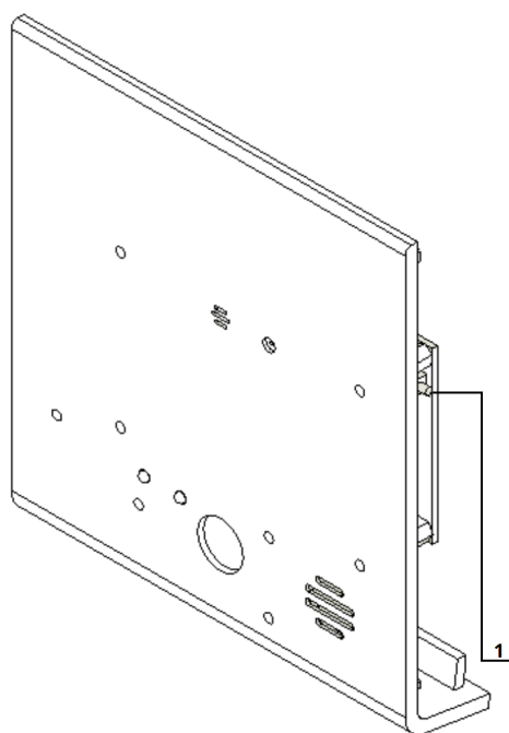
Рисунок 3 - Общий вид со снятой крышкой
