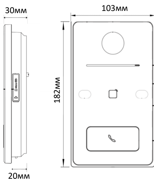
Вызывная панель
