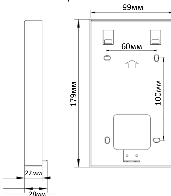
Монтажная коробка
