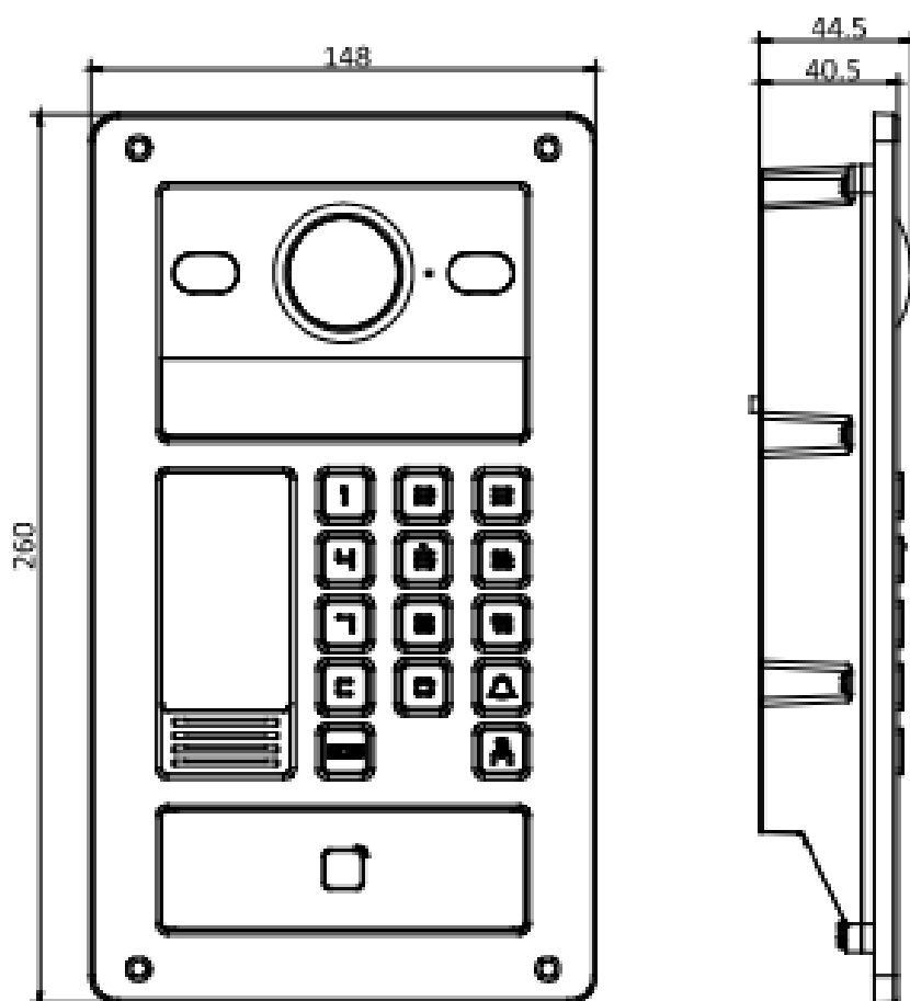
Габаритные размеры
