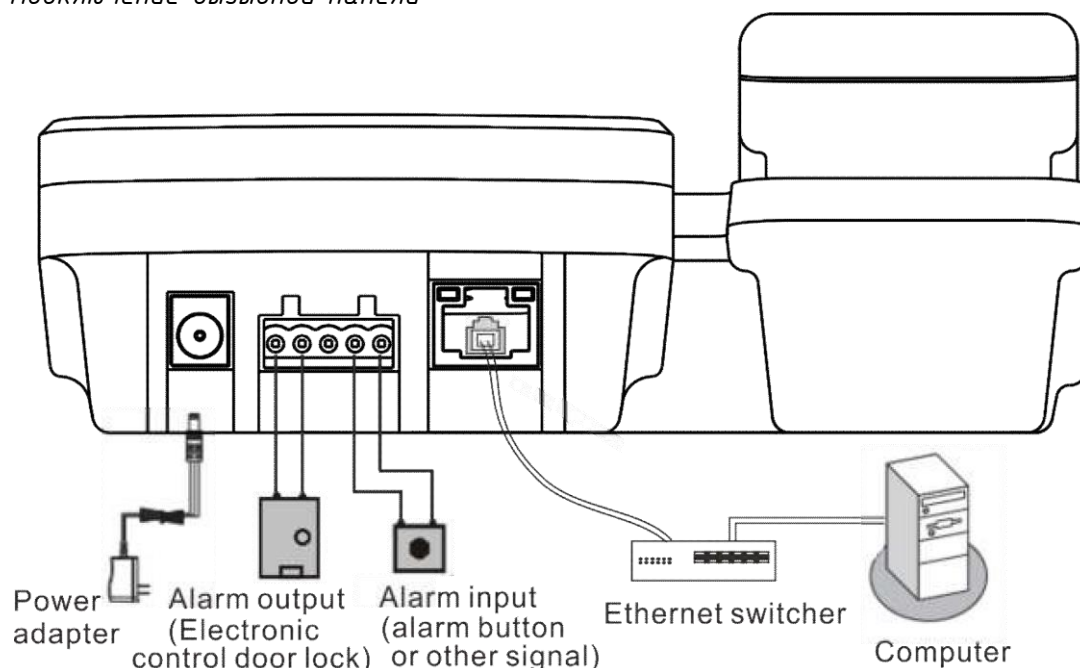
Подключение вызывной панели
