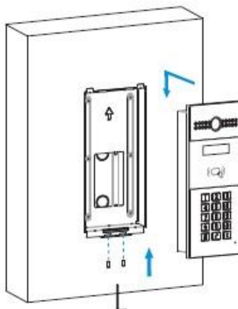
Установка в стену (заподлицо)
