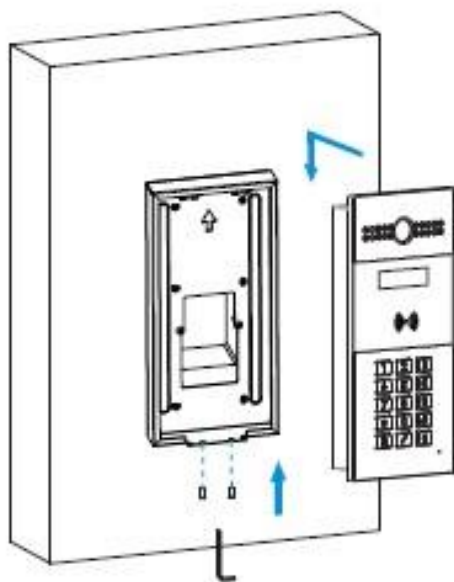
Установка на стену
