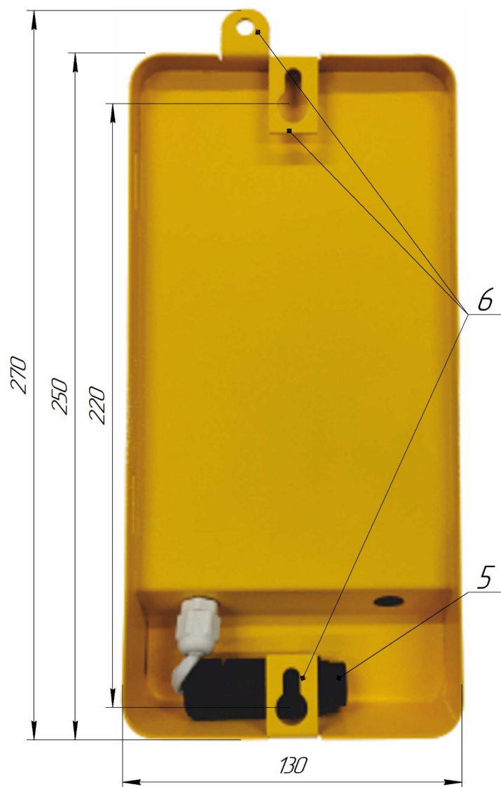
Рисунок 2 - Вид сзади
