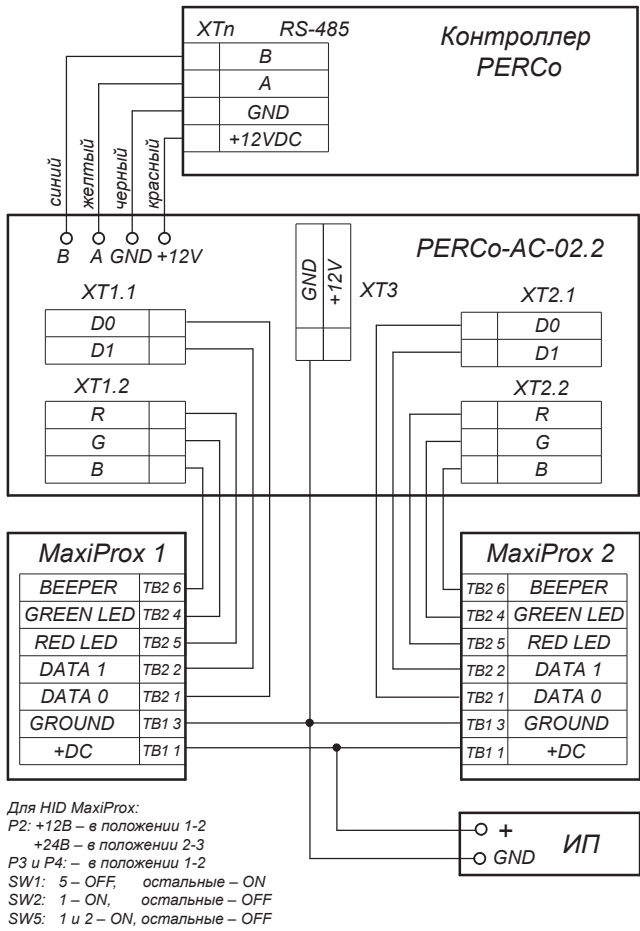
Пример подключения считывателя увеличенной дальности
