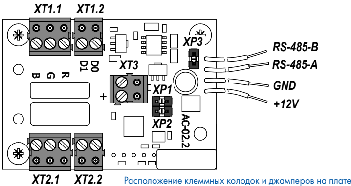
Расположение клеммных колодок и джамперов на плате
