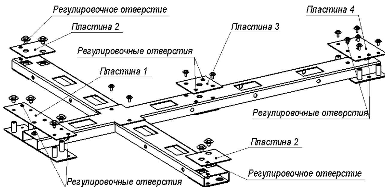
Рисунок 2. Схема сборки рамы.
