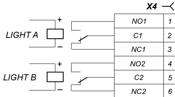
Рисунок 12. Выходные каскады для Light A и Light B
