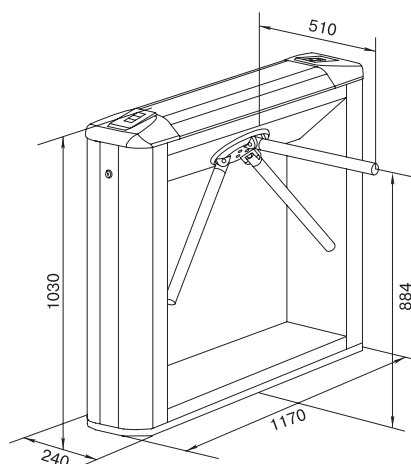
Габаритные размеры турникета PERCo-TB01.9A
