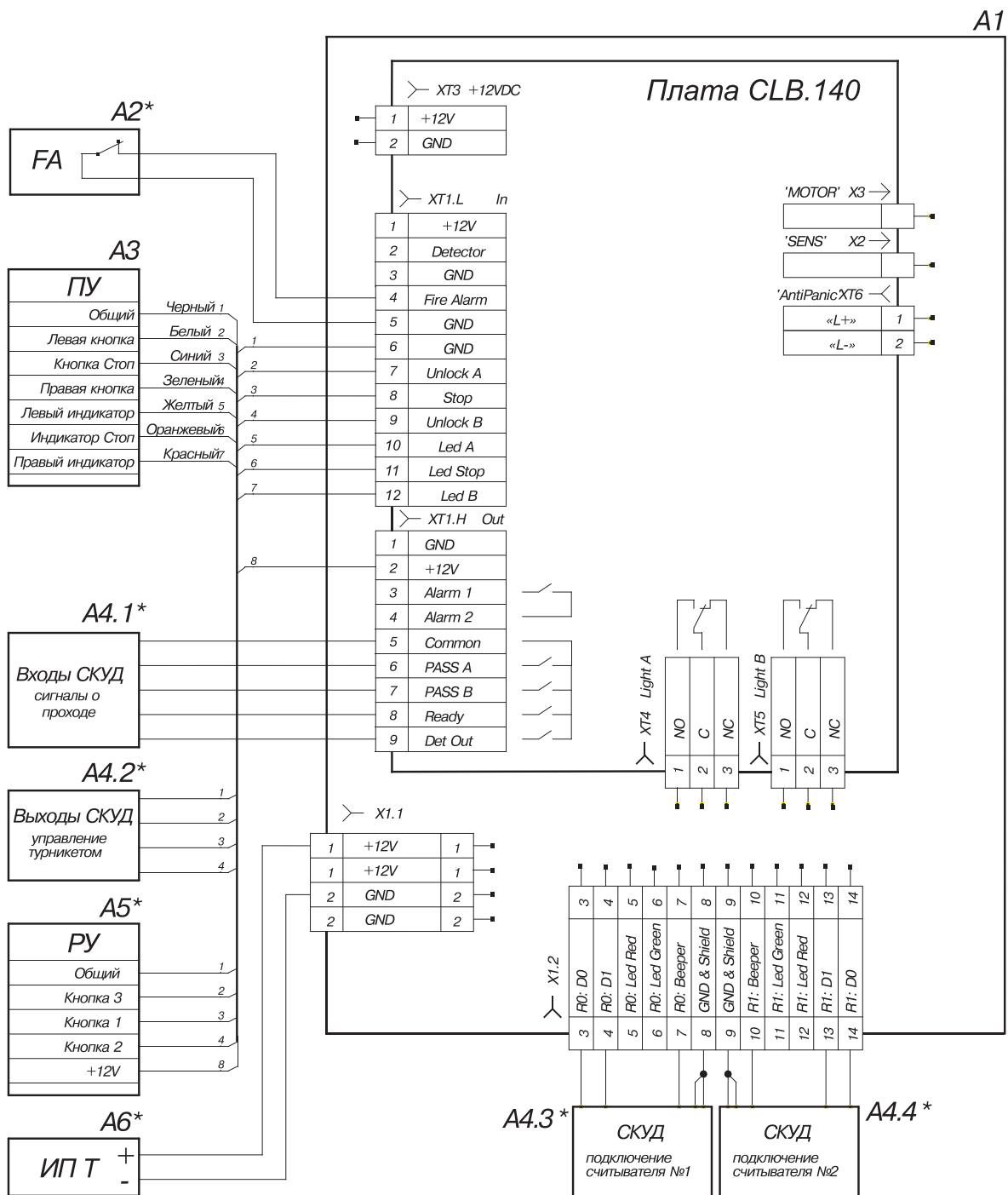
Схема соединений турникета PERCo-TV01.9А и дополнительного оборудования
