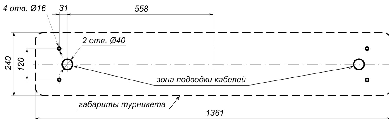
Рисунок 16. Схема разметки для установки стойки турникета 1
