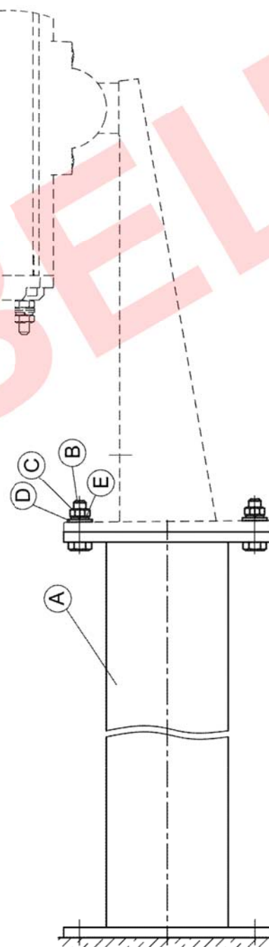
Рис.1 Установка переходника кронштейна ПК-200, -400, -600, -800, -1000
