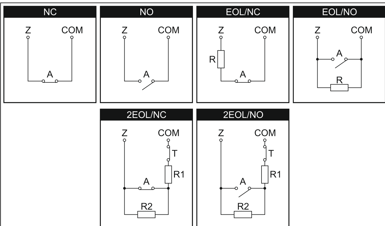
Рис. 9. Способы подключения извещателей к зонам. Контакты извещателя, обозначенные буквами: А - тревожные, Т – тамперные.
