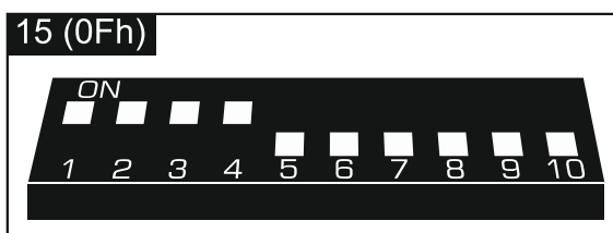
Рис. 8. Способ установки DIP-переключателей в модуле INT-O.
