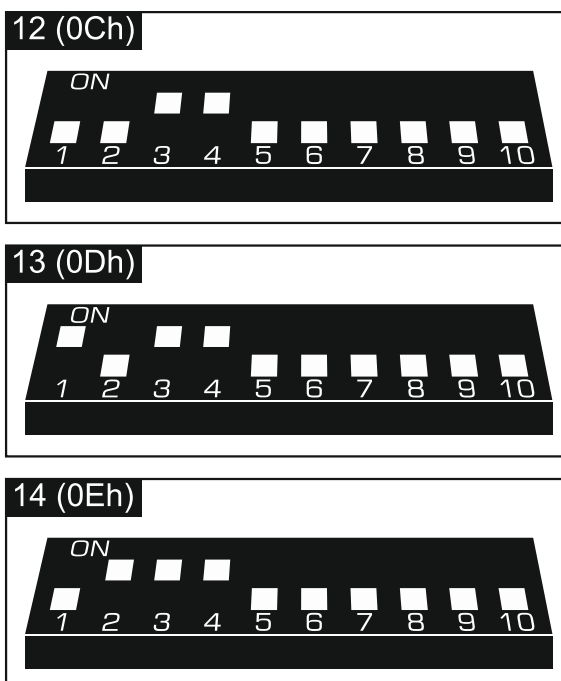
Рис. 6. Способ установки DIP-переключателей в модуле INT-E.
