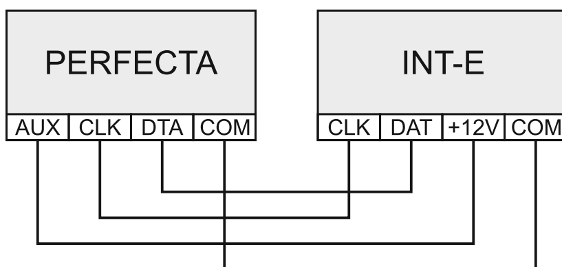
Рис. 5. Способ подключения модуля расширения INT-E к прибору.
