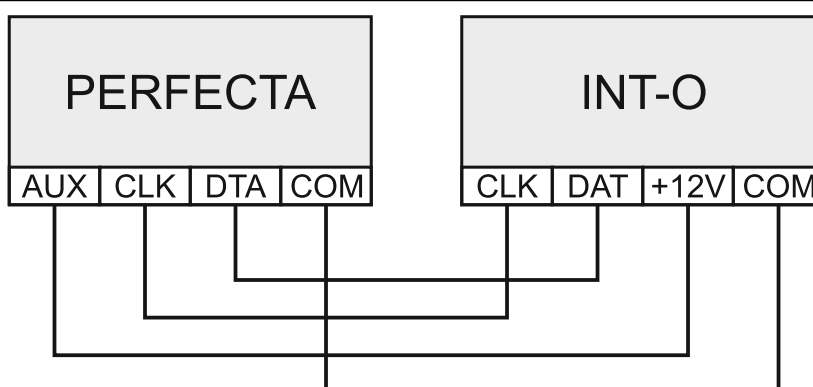
Рис. 7. Способ подключения модуля расширения INT-O к прибору.
