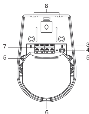
Рисунок 2 – Конструкция «Пирон-4 RED»
