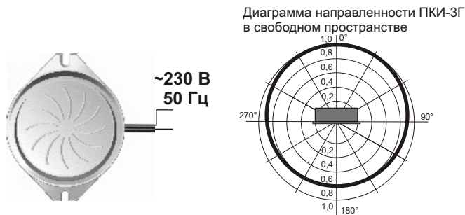
Рис.2 Схема подключения и диаграмма направленности оповещателя ПКИ-ЗГ.
