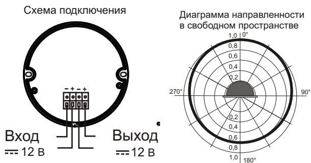
Рис.2 Схема подключения и диаграмма направленности оповещателя.
