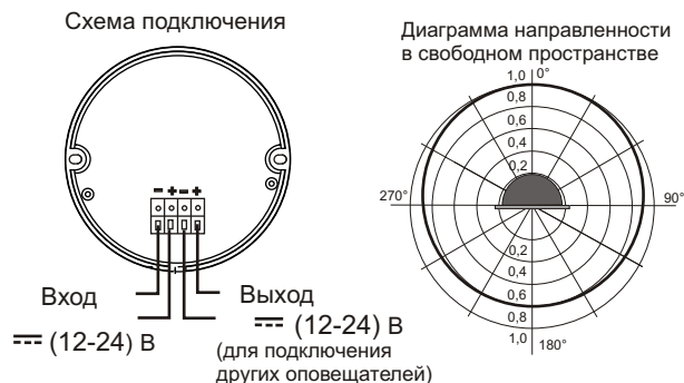
Рис.2 Схема подключения и диаграмма направленности оповещателя .
