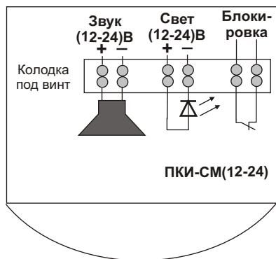
Рис.2 Схема подключения ПКИ-СМ(12-24).
