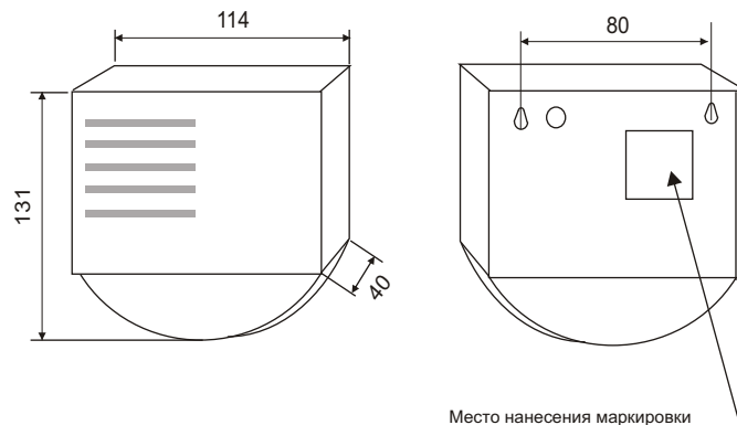
Рис.1. Габаритные, установочные размеры и эксплуатационное положение оповещателя.
