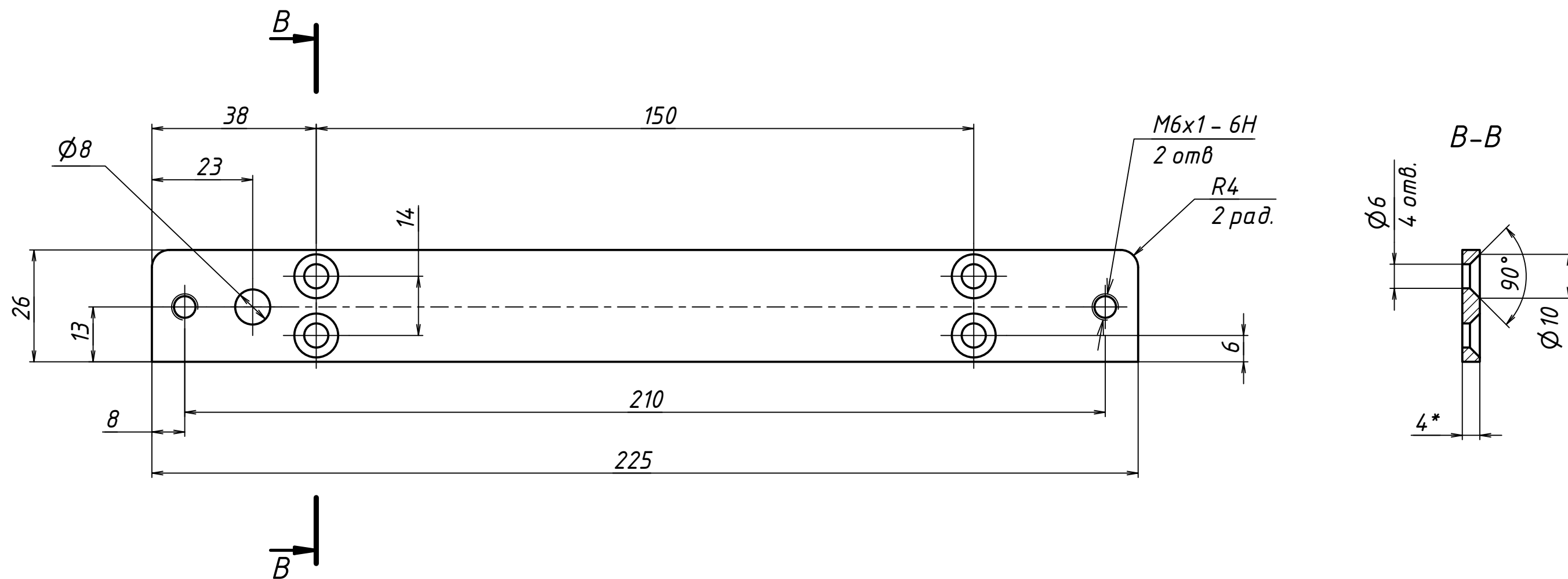
Габаритный чертеж Планка 400FP
