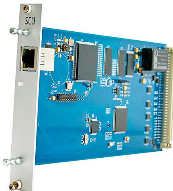
Рисунок 1 – Центральная плата SCU
