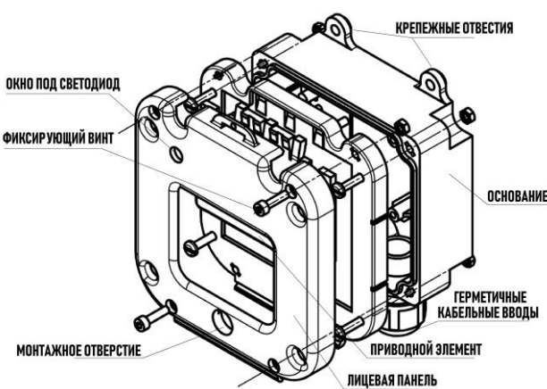
Рис.1. Элементы конструкции извещателя
