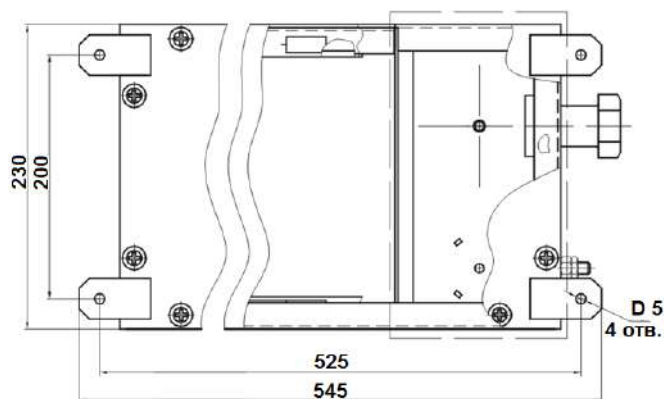
Рисунок 2 – Габаритные и посадочные оповещателя «Плазма»Ех(м) -40х20
