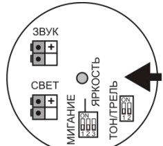
Рис.3 – Расположение клеммников и микропереключателей в коммутационном отсеке оповещателей «Плазма»Ех(м)-С3-40х20
