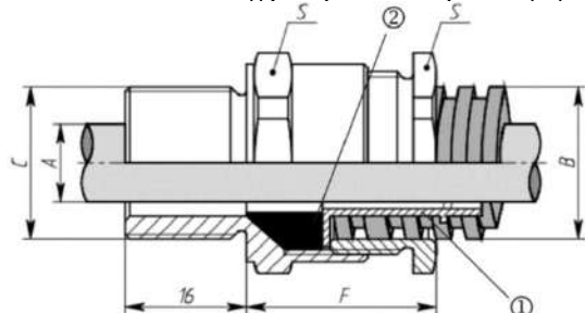
Рисунок 1 – Вариант герметичного кабельного ввода универсального взрывозащищённого.
