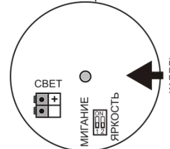
Рисунок 4 – Расположение клеммников и микропереключателей в коммутационном отсеке оповещателя «Плазма»Ex(m) - C
