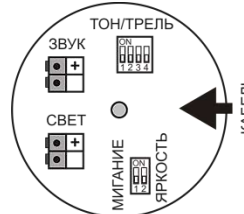
Рисунок 3 – Расположение клеммников и микропереключателей в коммутационном отсеке оповещателя «Плазма»Ex(m)–С3
