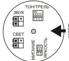
Рис.3 - Расположение клеммников и микропереключателей в коммутационном отсеке оповещателя «Плазма»Ex(m)-C3
