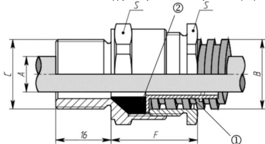
Рис. 1 – Вариант герметичного кабельного ввода универсального взрывозащищённого.
