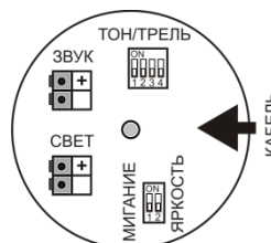
Рис.3 Расположение клеммников и микропереключателей в отсеке коммутационного оповещателя «Плазма»Ех- С3
