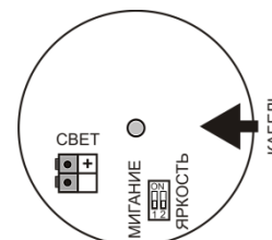
Рис.4 Расположение клеммников и микропереключателей в отсеке коммутационного оповещателя «Плазма»Ех - С
