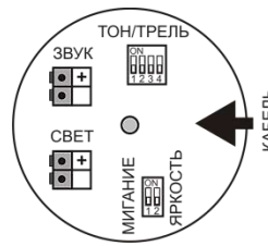
Рисунок 4 – Расположение клеммников и микропереключателей в коммутационном отсеке оповещателя «Плазма»Ех-СЗ
