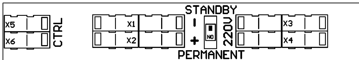
Рис.7 Расположение клеммных зажимов светильника
