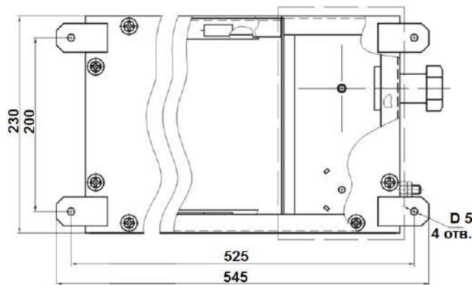
Рисунок 2 – Габаритные и посадочные оповещателя «Плазма»П220-40х20
