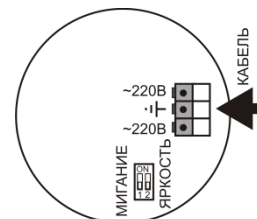
Рисунок 4 – Расположение клеммников и микропереключателей в коммутационном отсеке оповещателя «Плазма»П220 – С-40х20
