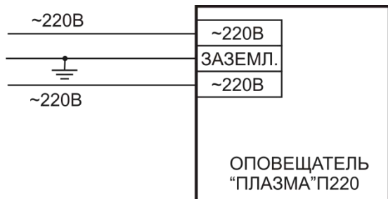
Рисунок 1 – Подключение оповещателя «Плазма»П220-40х20 к источнику питания 220В/50Гц.
