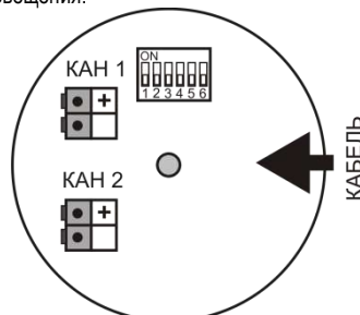
Рисунок 6 – Расположение клеммников и микропереключателей в коммутационном отсеке оповещателя «Плазма»П-С-40х20-2К.
