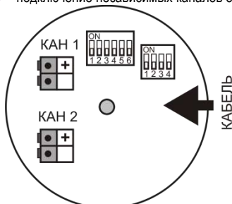
Рисунок 5 – Расположение клеммников и микропереключателей в коммутационном отсеке оповещателя «Плазма»П-С3-40х20-2К.
