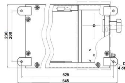
Рисунок 2 – Габаритные и посадочные оповещателя «Плазма»П-40х20-2К
