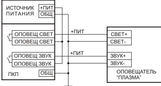
Рисунок 2 – Подключение оповещателя «Плазма»П-40х20 к релейным каналам оповещения приёмно-контрольного прибора.
