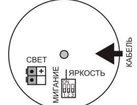
Рисунок 5 – Расположение клеммников и микропереключателей в коммутационном отсеке оповещателей «Плазма»П – С-40х20
