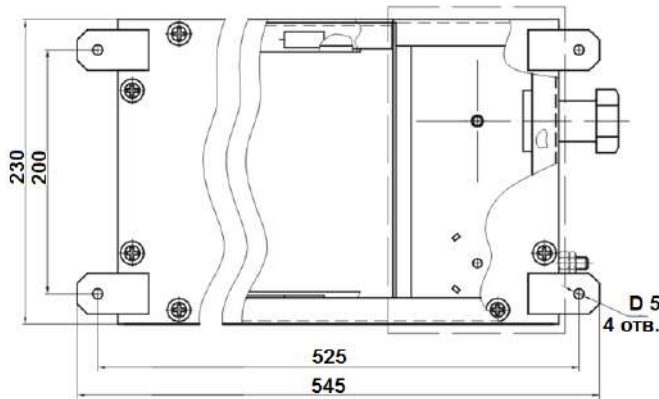
Рисунок 3 – Габаритные и посадочные оповещателя «Плазма»П-40х20
