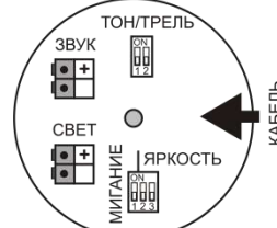
Рисунок 4 – Расположение клеммников и микропереключателей в коммутационном отсеке оповещателей «Плазма»П- С3-40х20
